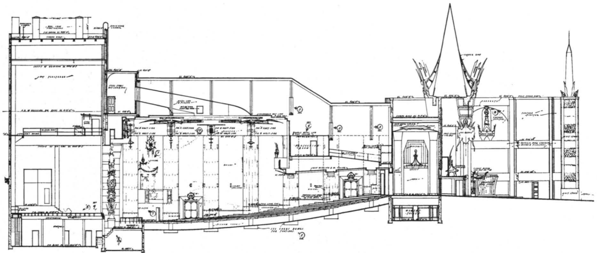
LONGITUDINAL SECTION
